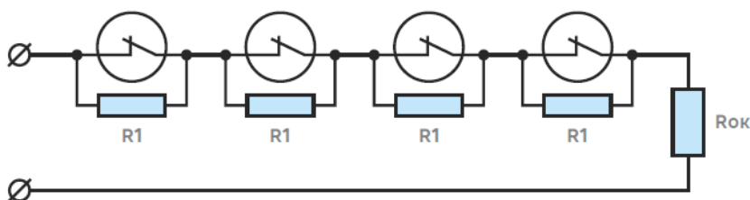
Рис.3. Схемы подключения к шлейфу сигнализации КТМ охранных или контрольных извещателей. Номиналы резисторов ( \pm 5\% ): R_{ок} = 560 \text{ Ом} ; R1 = 2,2 \text{ кОм} .
